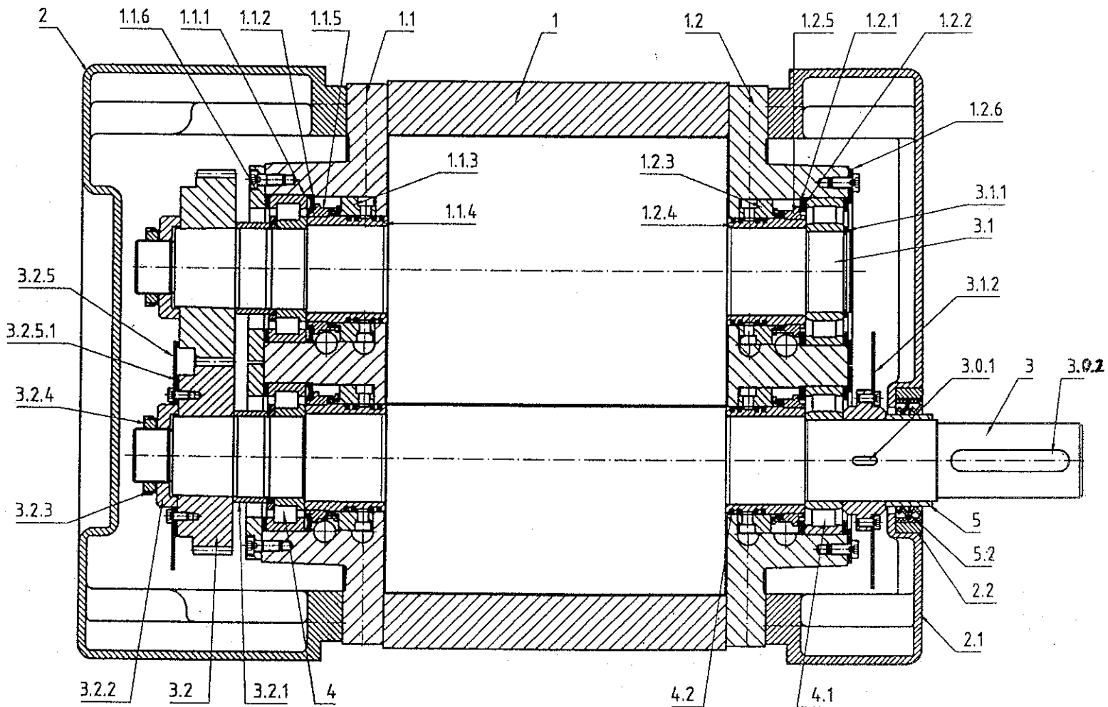
Drehkolben Verdichter Schnittzeichnung 3 RV
